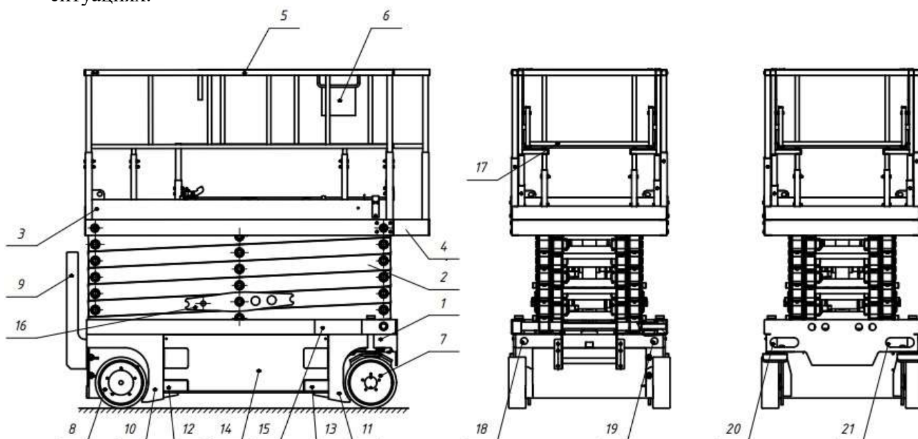
Рисунок 2 – Общий вид подъемника с рабочей платформой
