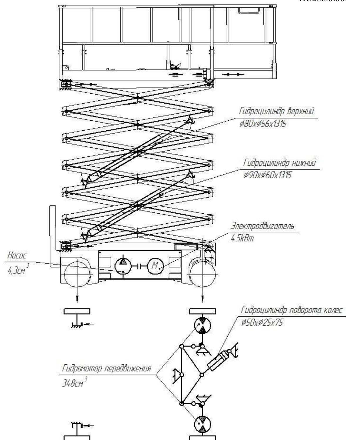
Рисунок Б2 – Кинематическая схема подъемников с рабочей платформой ЭКО12 ПСП-1062.11,5ПС25, ЭКО14 ПСП-1062.13,5ПС26, ЭКО16 ПСП-1062.15,5ПС26**
