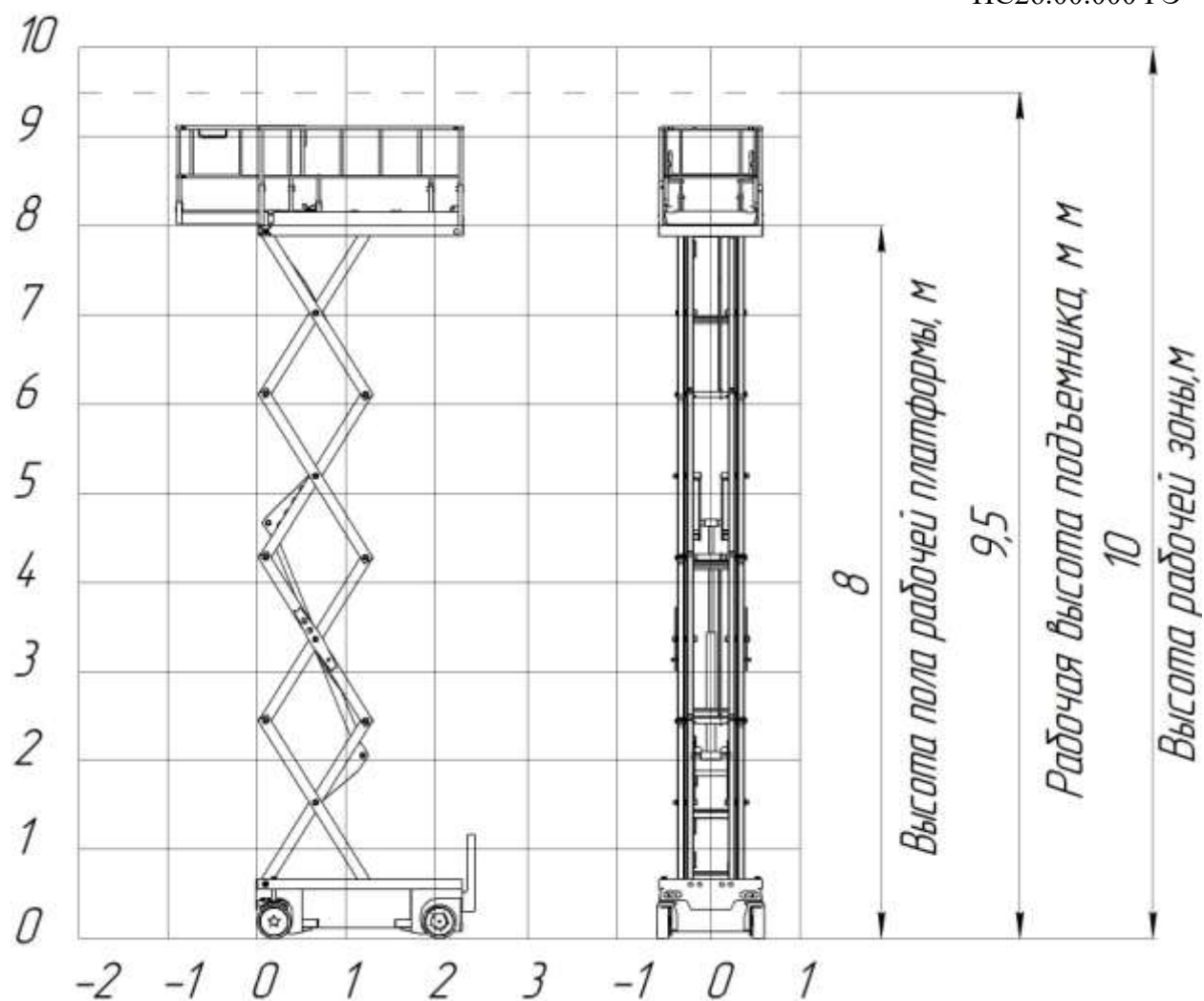
Рисунок А2 – Высотные характеристики подъемника с рабочей платформой ЭКО10 ПСП-1062.9,5ПС24 ТУ4837-001-68138980-2016
