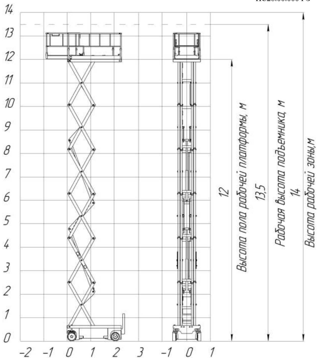
Рисунок А4 – Высотные характеристики подъемника с рабочей платформой ЭКО14 ПСП-1062.13,5ПС26 ТУ4837-001-68138980-2016
