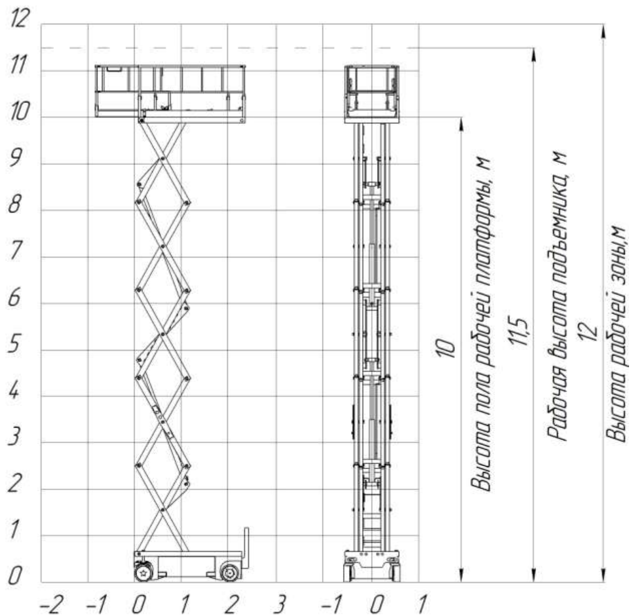
Рисунок А3 – Высотные характеристики подъемника с рабочей платформой ЭКО12 ПСП-1062.11,5ПС25 ТУ4837-001-68138980-2016
