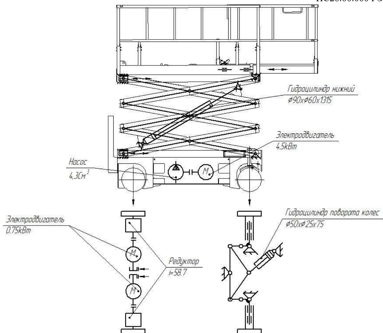
Рисунок Б3 – Кинематическая схема подъемников с рабочей платформой ЭКО8 ПСП-1062.7,5ПС23, ЭКО10 ПСП-1062.9,5ПС24*
