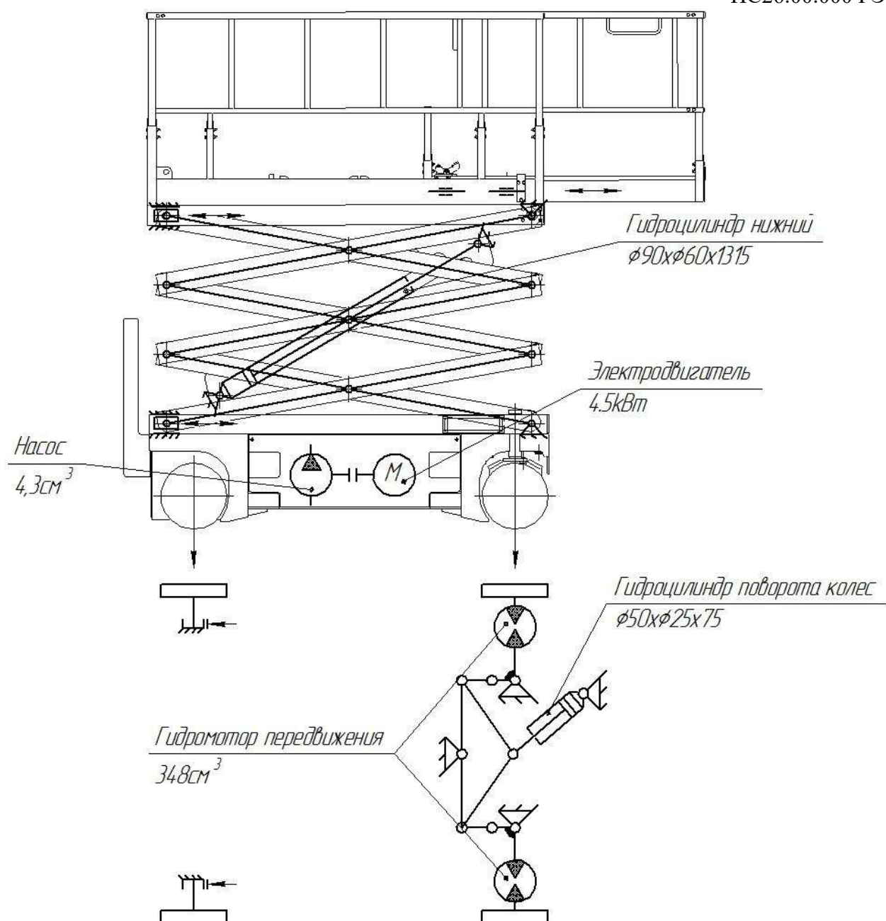
Рисунок Б4 – Кинематическая схема подъемников с рабочей платформой ЭКО8 ПСП-1062.7,5ПС23, ЭКО10 ПСП-1062.9,5ПС24**
