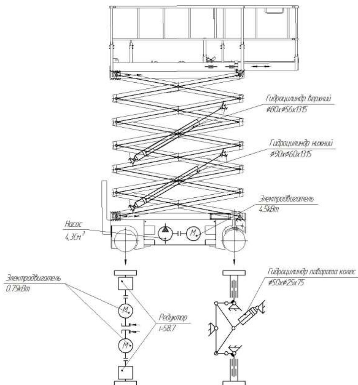
Рисунок Б1 – Кинематическая схема подъемников с рабочей платформой ЭКО12 ПСП-1062.11,5ПС25, ЭКО14 ПСП-1062.13,5ПС26, ЭКО16 ПСП-1062.15,5ПС26*
