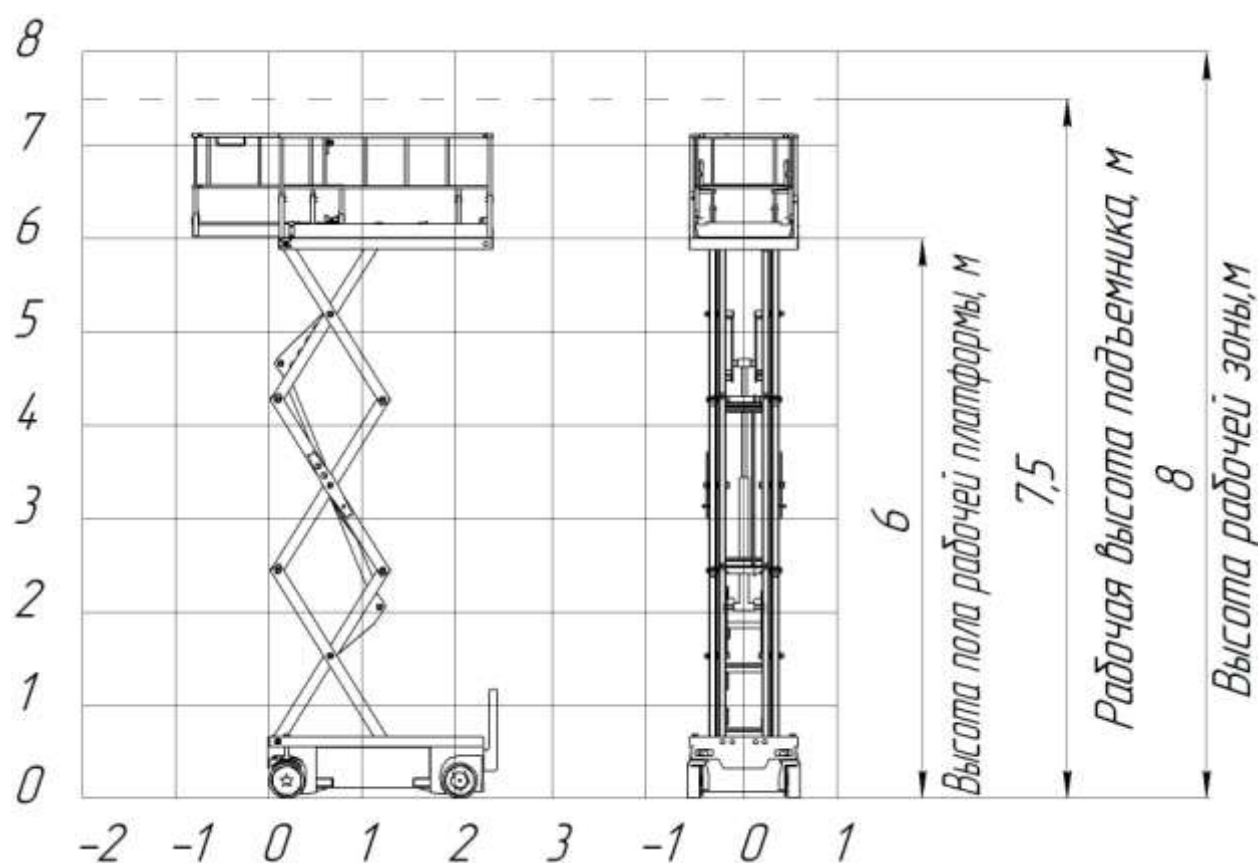
Рисунок А1 – Высотные характеристики подъемника с рабочей платформой ЭКО8 ПСП-1062.7,5ПС23 ТУ4837-001-68138980-2016
