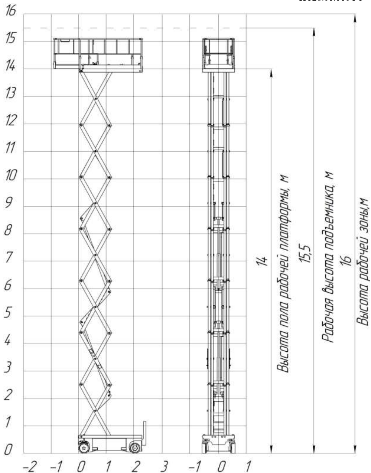
Рисунок А5 – Высотные характеристики подъемника с рабочей платформой ЭКО16 ПСП-1062.15,5ПС27 ТУ4837-001-68138980-2015
