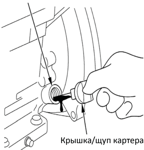
Маслозаливная горловина
