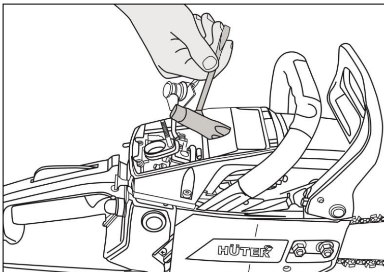
Рис. 37. Откручивание свечи
