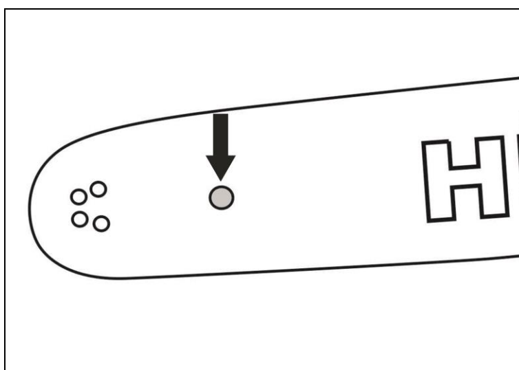
Рис. 28. Отверстие для смазки ведомой звездочки
